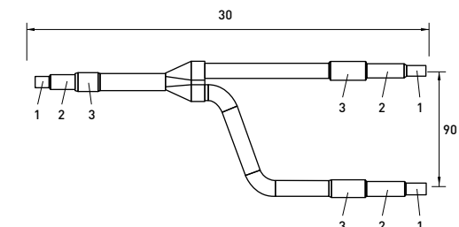
Flüssigkeitsleitung
