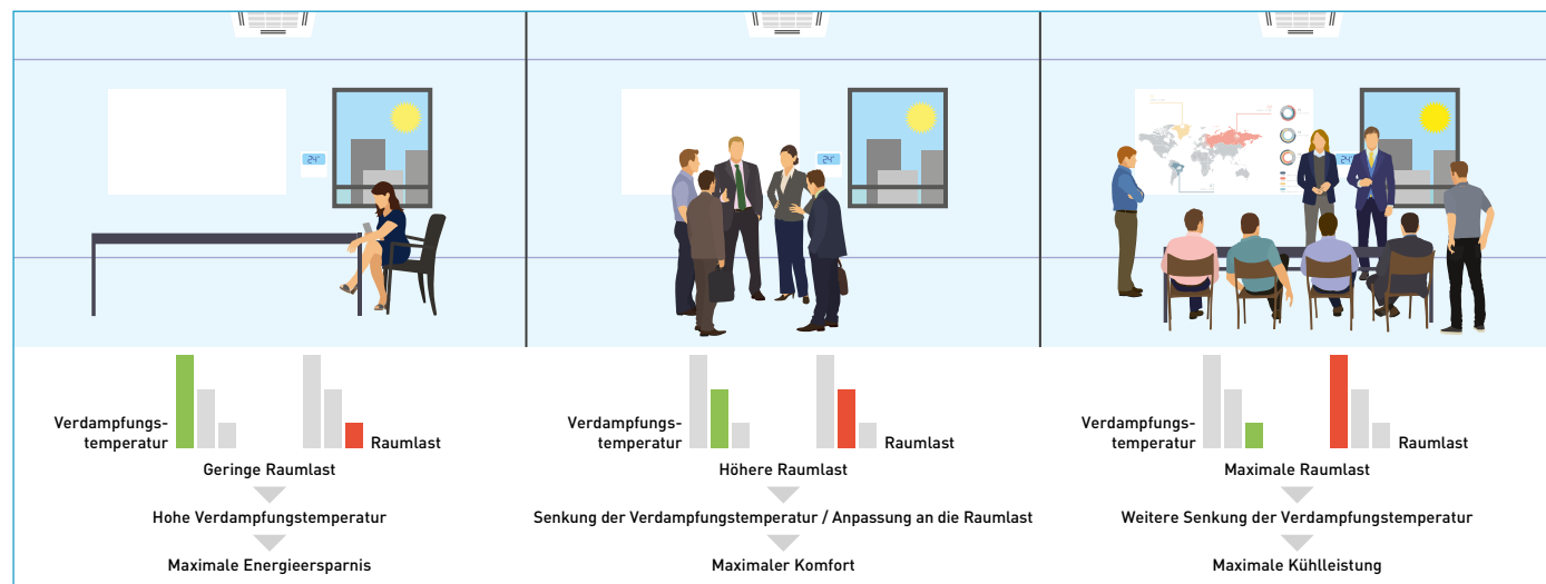
Lastabhängige, modulierende Regelung der Verdampfungstemperatur am Beispiel des Kühlbetriebs (für Heizbetrieb entsprechend)
